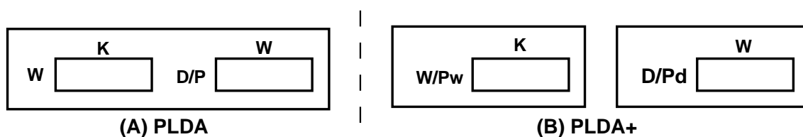
图 3.2 PLDA和PLDA+中文档和词项-主题矩阵的分配策略。
