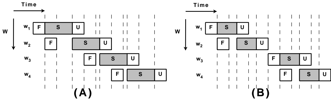
图 3.4 PLDA+中的流水线吉布斯采样策略。(A): t_s \geq t_f + t_u ; (B): t_s < t_f + t_u 。在该图中, F 表示获取主题分布信息操作(fetching), U 表示更新主题分布信息操作(updated), 而 S 表示采样操作(sampling)。
