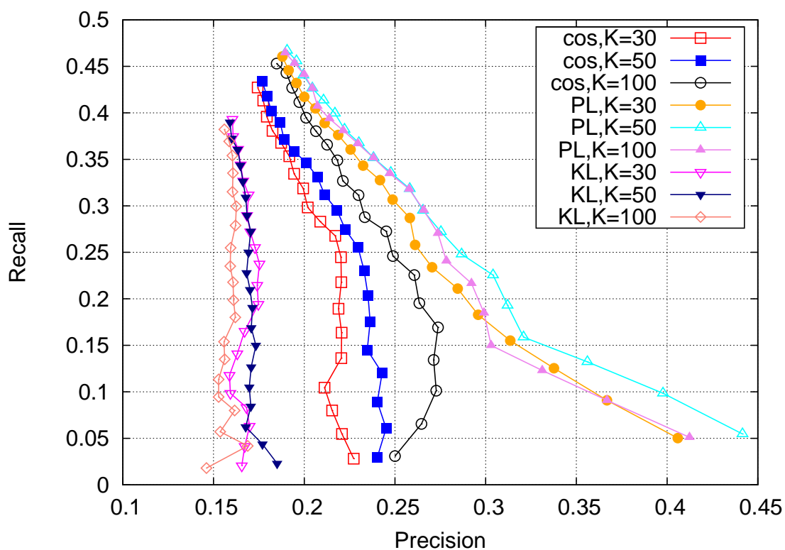
(a) 在NEWS数据集上学习LDA模型
