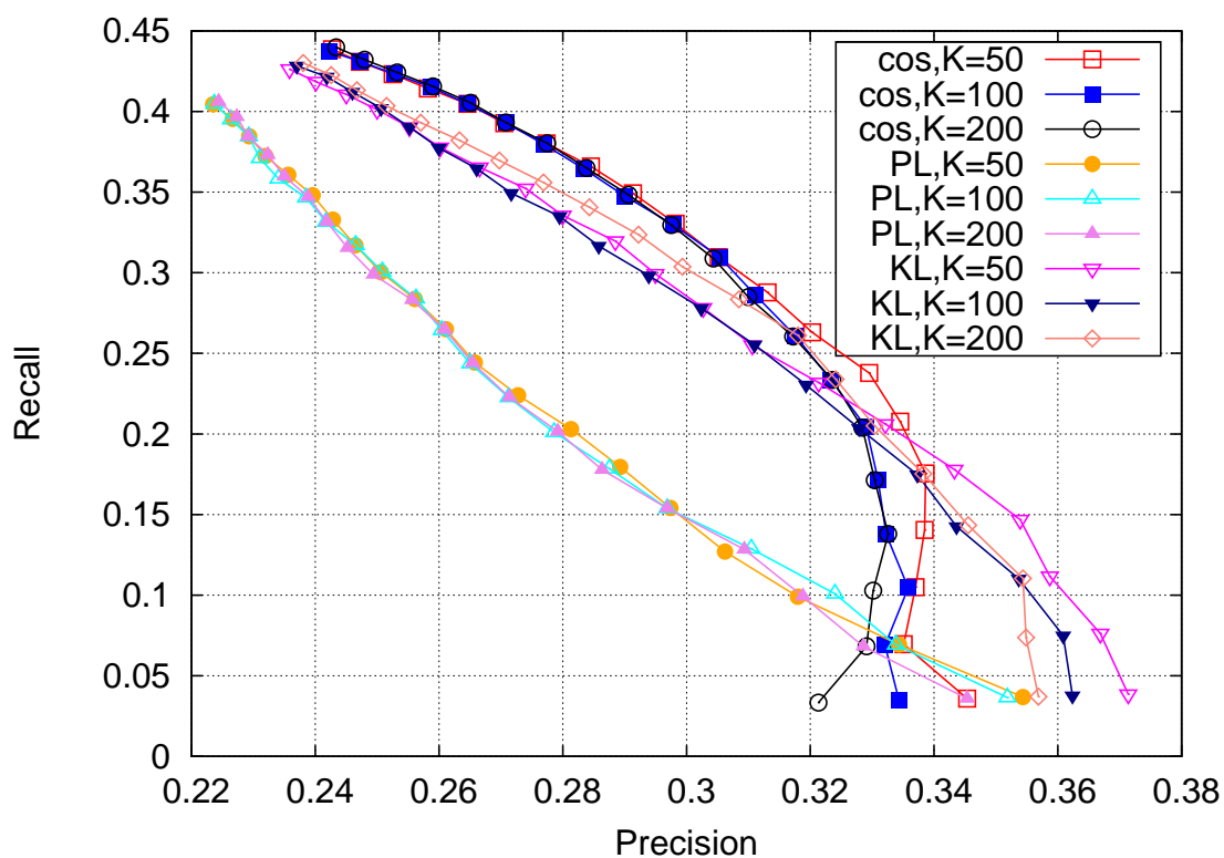
(a) 在RESEARCH数据集上学习LDA模型
