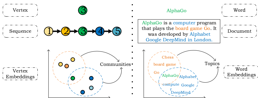
图 7.2 网络表示学习和文本建模之间的类比关系：网络中的节点、序列和社区分别对应文本中的词、文档和主题。
