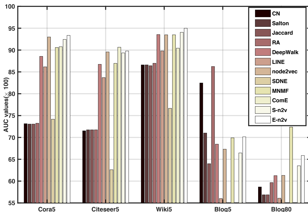
图 7.6 移除不同比例边后的链接预测结果
