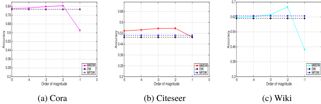
图 4.4 MMDW 在不同数据集上的参数敏感性分析
