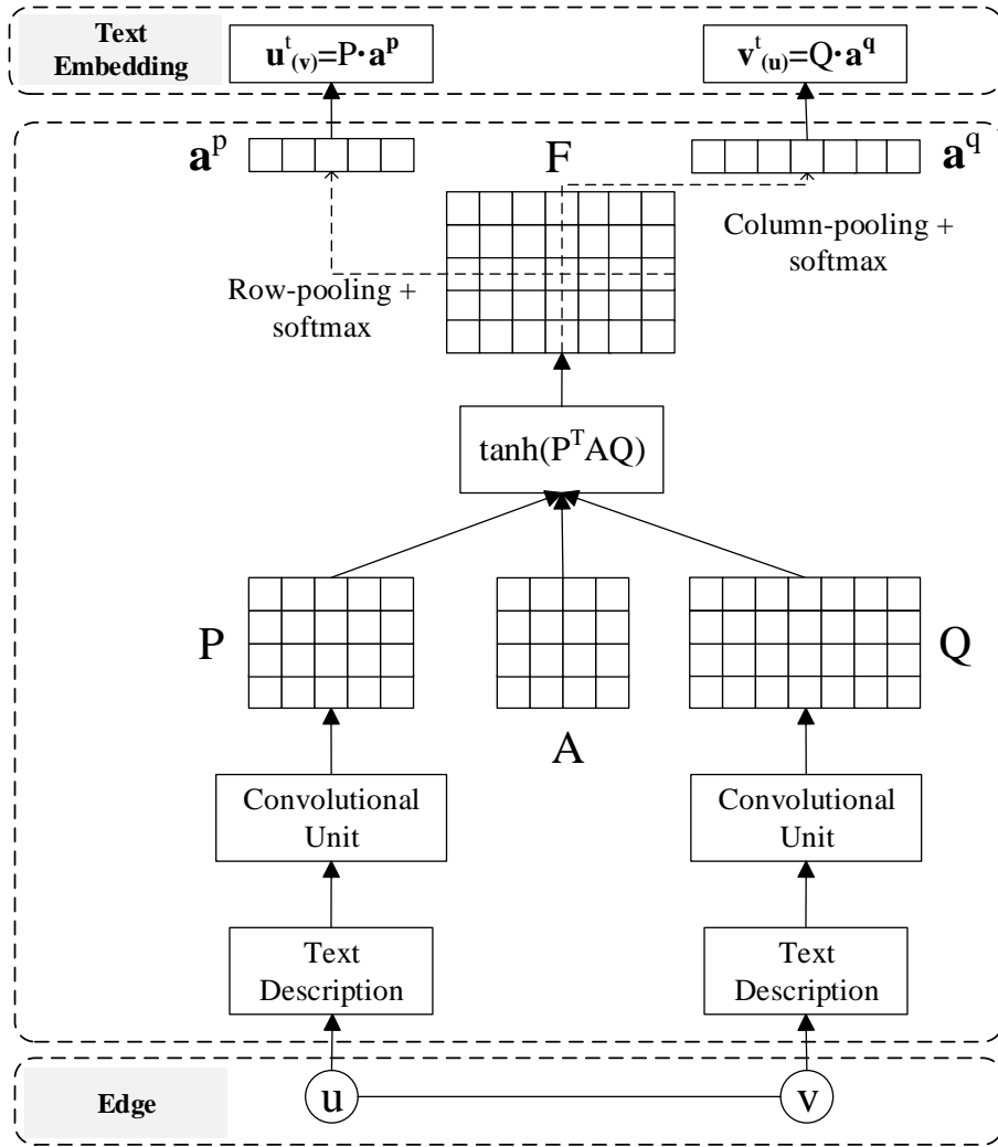
图 5.2 上下文相关文本表示示意图
