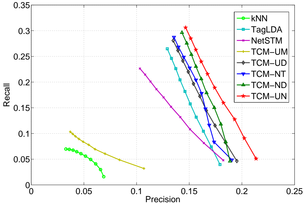
图 3.3 社会标签推荐结果
