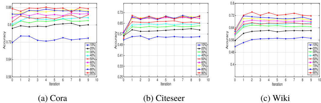
图 4.3 MMDW 在不同数据集上的收敛情况
