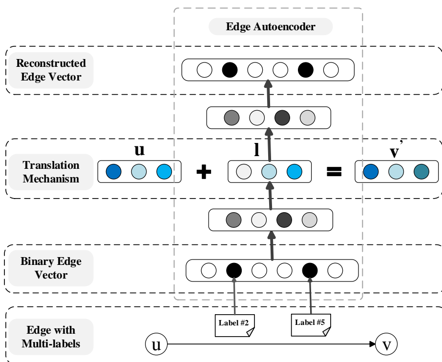
图 6.3 TransNet 模型示意图
