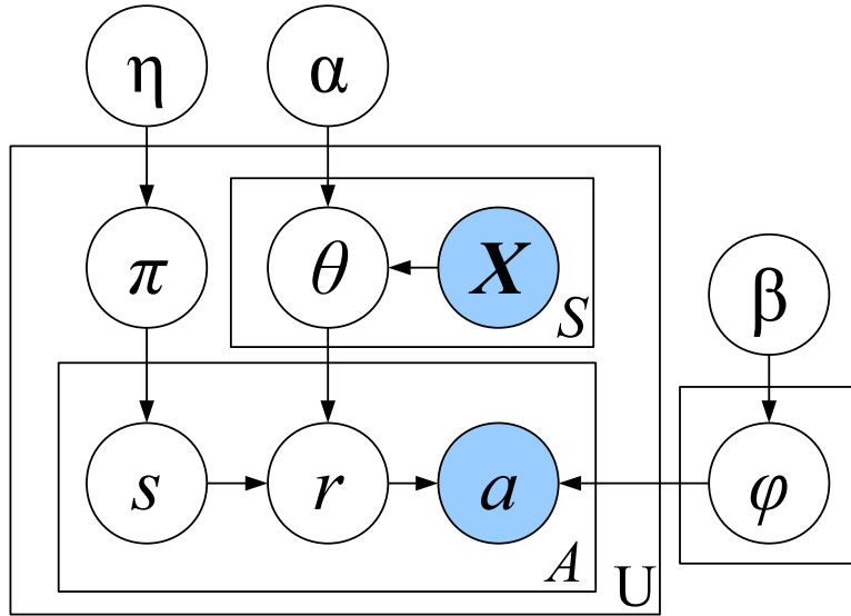
图 3.1 标签关联模型 (Tag Correspondence Model)
