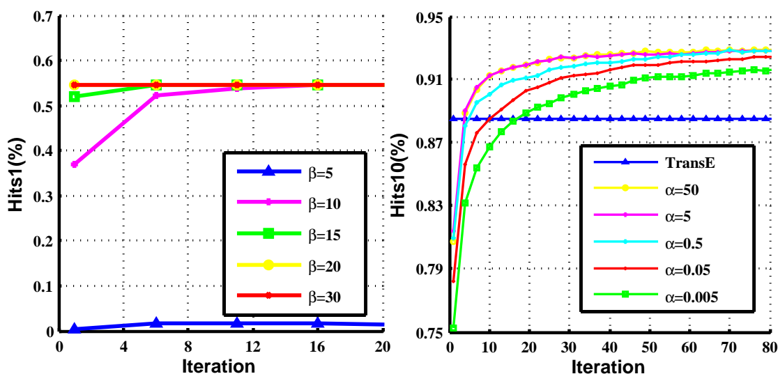
图 6.4 参数敏感性分析
