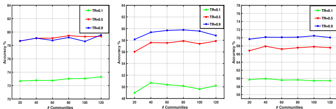
(a) Cora 上分类准确率 (b) Citeseer 上分类准确率 (c) Wiki 上分类准确率
