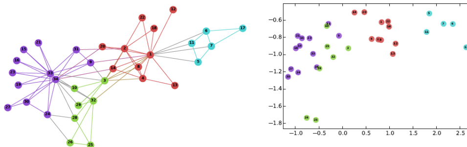
图 1.4 Karate 网络低维向量表示可视化 [1]
