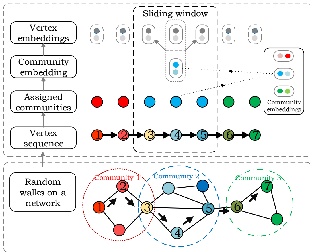
图 7.3 CNRL 模型示意图
