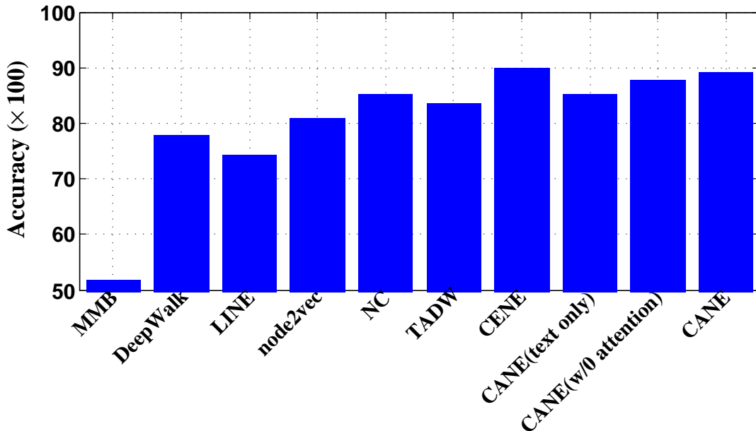
图 5.3 Cora 数据集节点分类结果
