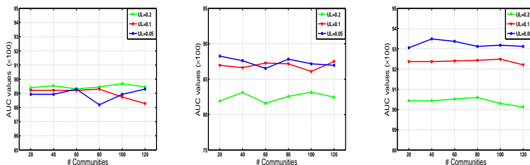
(a) Cora 上的 AUC 结果 (b) Citeseer 的 AUC 结果 (c) Wiki 的 AUC 结果
